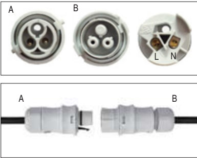
Completo di connettore IP68 per una rapida installazione - Complete with IP68 connector for quick installation
