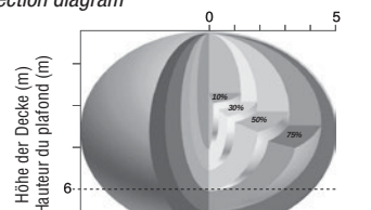
Erfassungsschema für die Deckmontage (m) Schéma de détection plafond (m)
