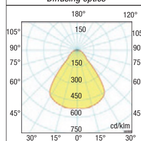
Ottica diffusante Diffusing optics
