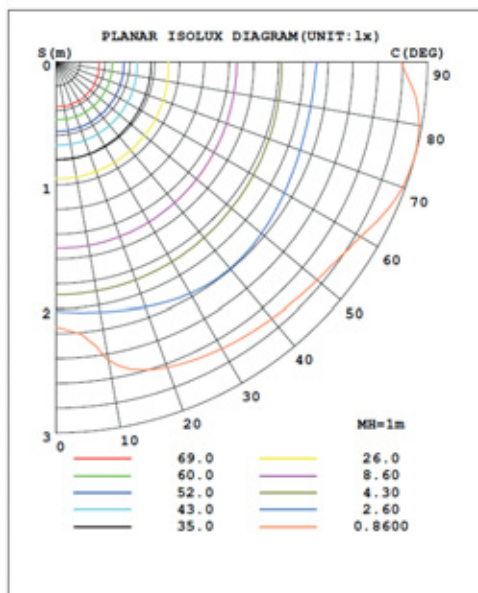
AREA APERTA LENTE SIMMETRICA OPEN AREA SYMMETRIC LENS
