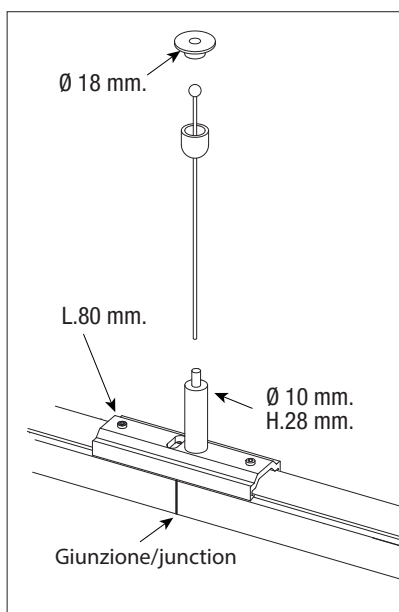
Kit sospensione con staffa lunga e tenditore automatico per giunzione fila continua, cavo 3m in acciaio Ø 1,5 mm. Suspension kit with long bracket and automatic gripper for continuous row junction, 3m cable in steel Ø 1.5 mm.
