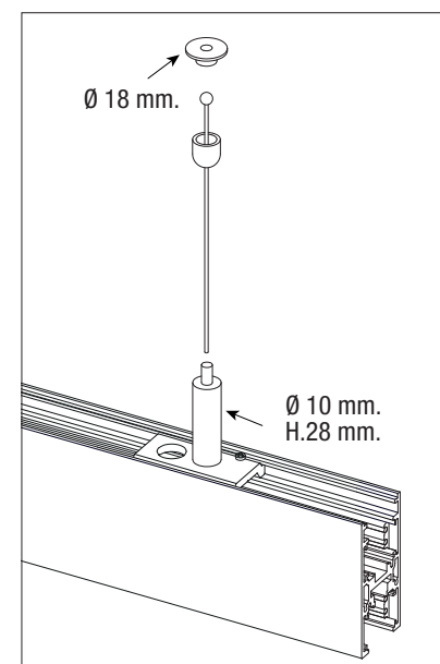
Kit sospensione con staffa corta e tenditore automatico, cavo 3m in acciaio Ø 1,5 mm. Suspension kit with short bracket and automatic gripper, 3m cable in steel Ø 1.5 mm.
