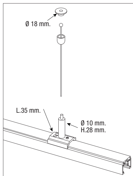
Kit sospensione con staffa corta e tenditore automatico, cavo 3m in acciaio Ø 1,5 mm. Suspension kit with short bracket and automatic gripper, 3m cable in steel Ø 1.5 mm.
