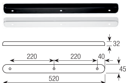
ROSONE RETTANGOLARE 3 FORI RECTANGULAR CEILING ROSE - 3 HOLES
