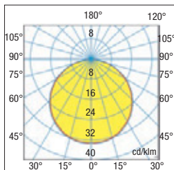
Dati fotometrici Photometric data
