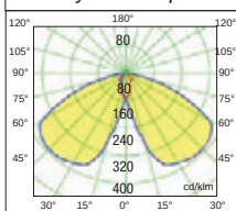
Ottica bi-asimmetrica bi-asymmetric optics
