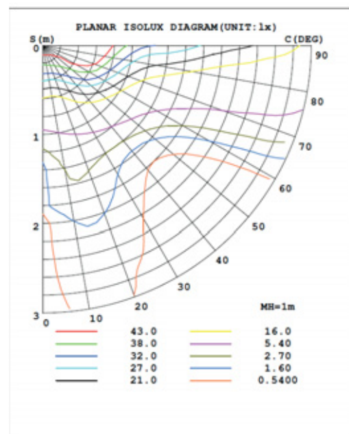
LENTE per CORRIDOIO LENTE ASIMMETRICA CORRIDOR LENS ASYMMETRIC LENS
