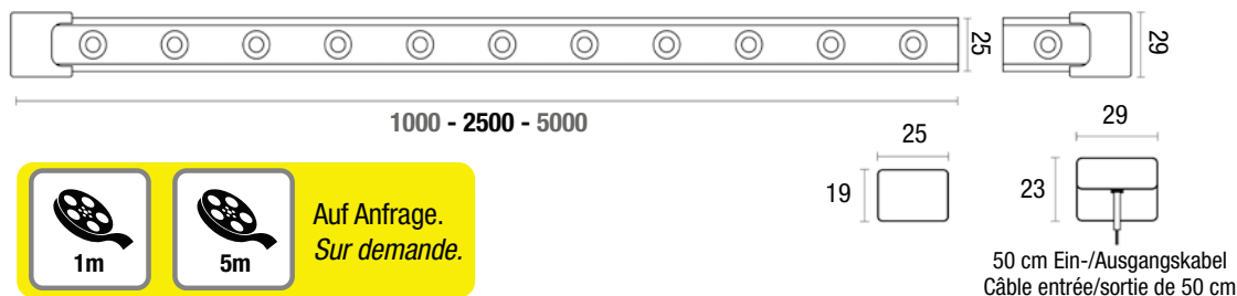
RE-FL129-1 1 Meter Aluminiumprofil. Profilé aluminium de 1 mètre.
