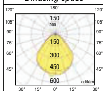
Ottica diffondente Diffusing optics
