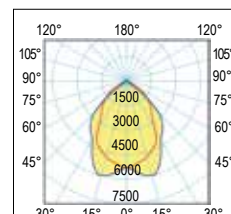
90° Diffondente - Wide
