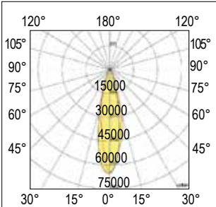
25° Concentrante - Spot
