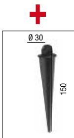
Cod. 24165 Picchetto in alluminio Aluminum picket
