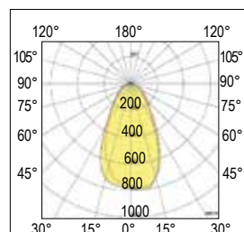
60° Diffondente - Flood
