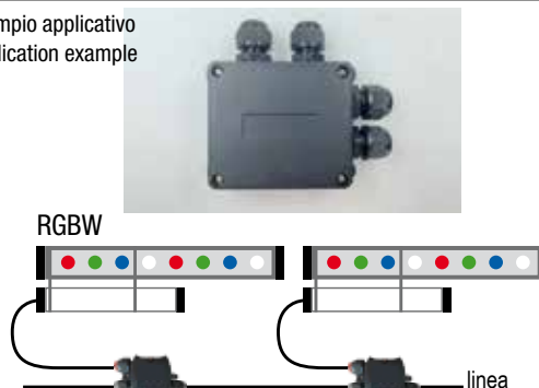
Cod. XPG9-P104 Accessorio IP67 per linee di luce continua IP67 accessory for continuous light lines.
