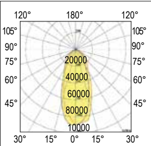
40° - Semi-diffondente - Wide
