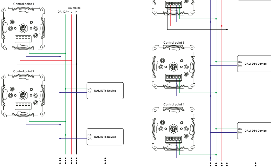
Schema di collegamento - Wiring diagram
