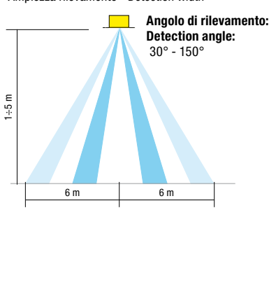
Ampiezza rilevamento - Detection width
