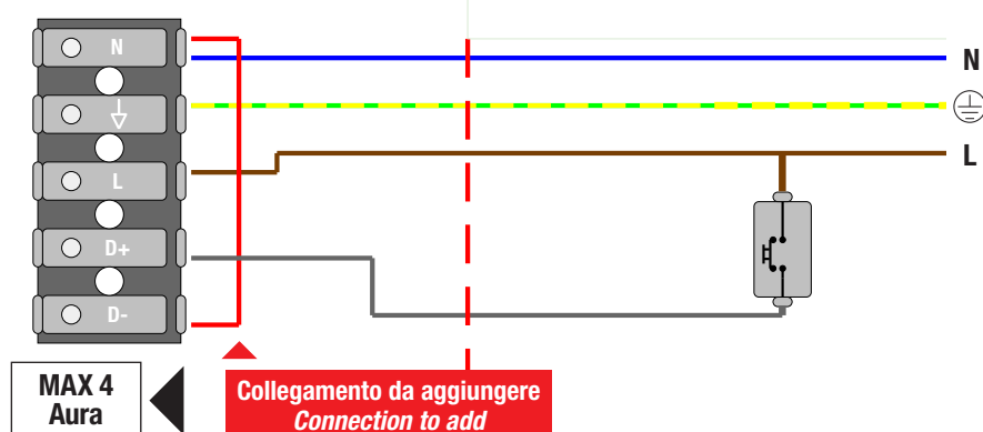
Regolazione a pulsante con driver Dali, impianto tradizionale + un filo Push button adjustment with Dali driver, traditional system + one wire
