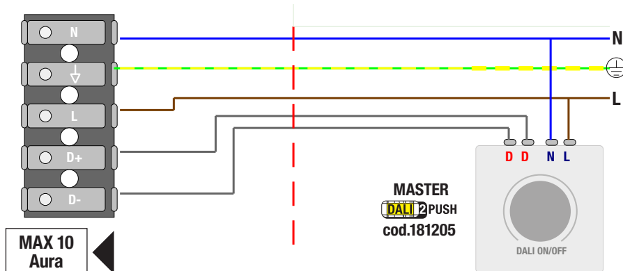
Regolazione Dali, impianto tradizionale + due fili Dali regulation, traditional system + two wires
