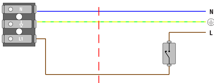
Accensione indipendente, impianto tradizionale + un filo Ø800, Ø1200. Independent ignition, traditional system + one wire Aura Ø800, Ø1200 and two rings (Ø400 + Ø600).
