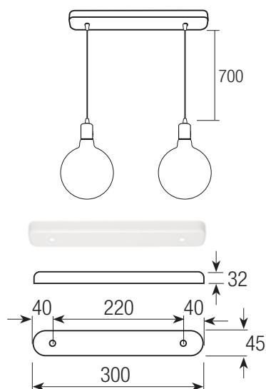
ROSONE RETTANGOLARE 2 FORI 2-HOLE RECTANGULAR CEILING ROSE
