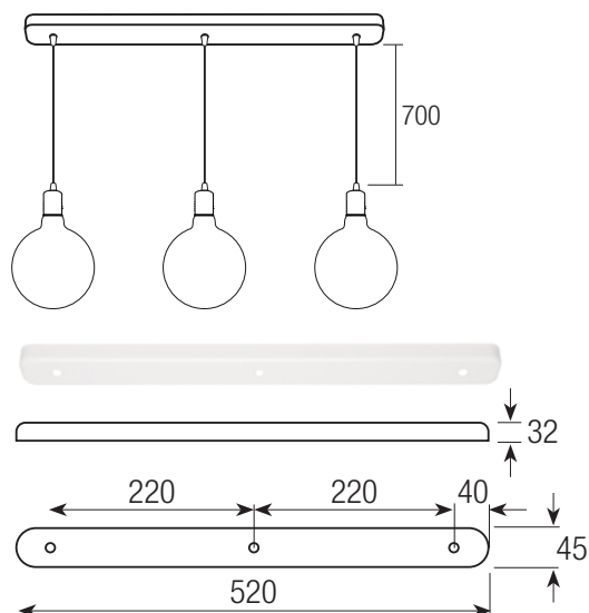
ROSONE RETTANGOLARE 3 FORI 3-HOLE RECTANGULAR CEILING ROSE
